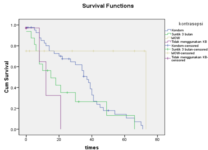
Gambar 1. Kaplan-Meier lama penggunaan kontrasepsi Wanita ODHA.
